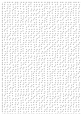
Slika 1: Shema neenakomerne računske mreže
